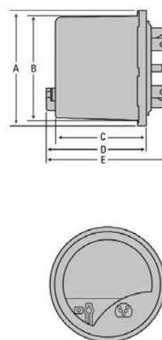
SENTINEL® Socket Meter
